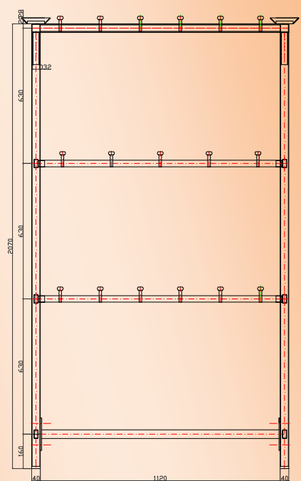
BASTIDOR 63 PIEZAS 4+3+4 BARRAS - 6+5+6 GANCHOS/BARRA BASTIDOR 68 PIEZAS 4+4+4 BARRAS - 6+5+6 GANCHOS/BARRA
